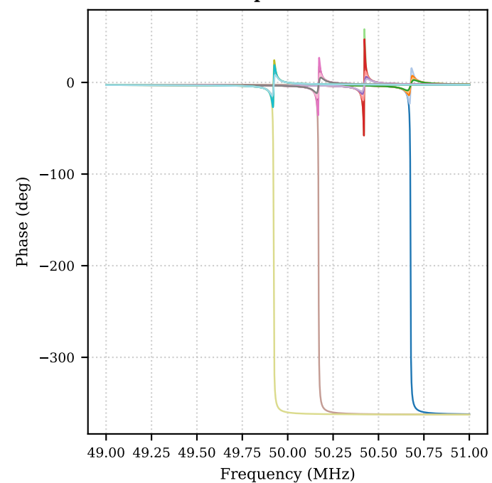
Cp = 300f
