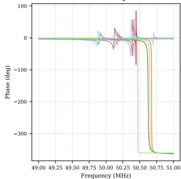
Itail = 975 \mu
